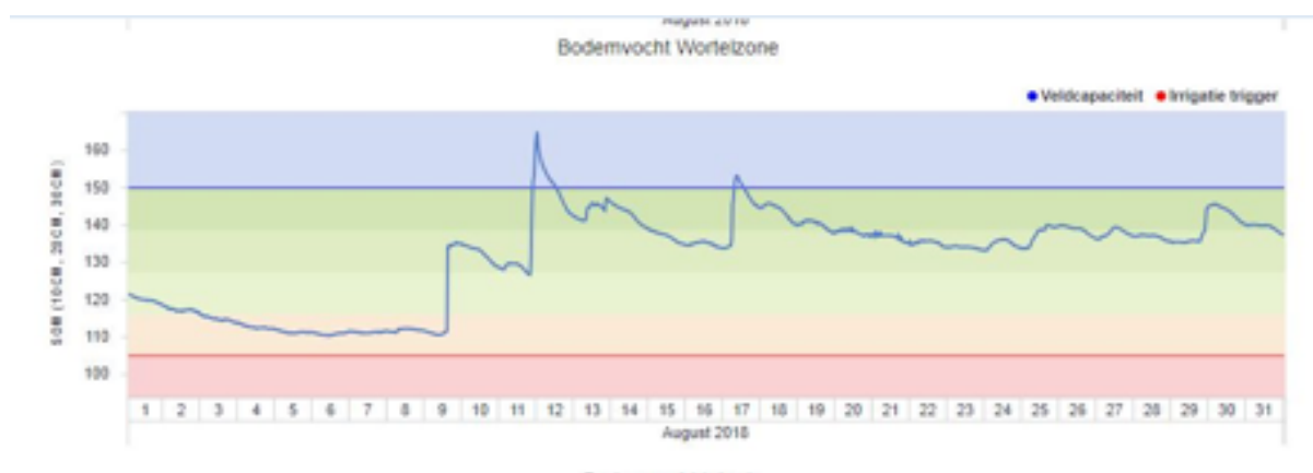
Figuur 4. Een voorbeeld van de data van een bodemvochtsensor.
